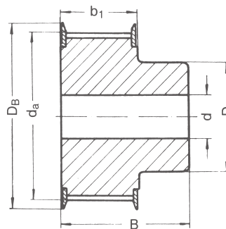
Ausführung ZBN
