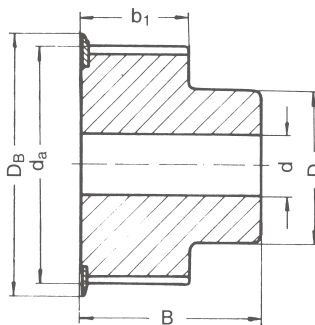
Ausführung EBN
