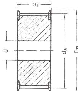
Ausführung ZB
