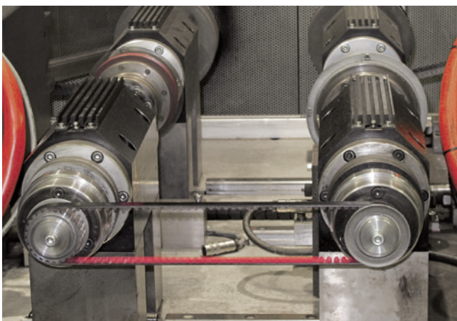
Abbildung 1.2.1: Prüfstand
