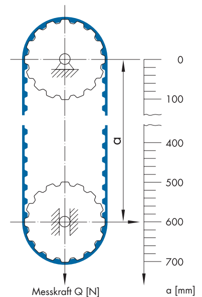
Abbildung 1.3.2: Anordnung zum Messen der Riemenlänge
