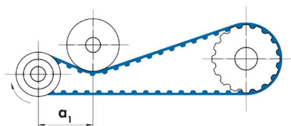
Abbildung 5.1.2: Anordnung der Außenspannrolle
