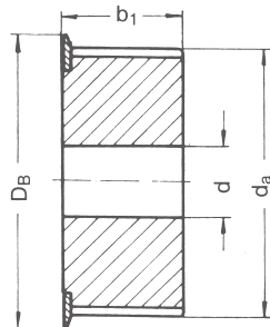
Ausführung EB
