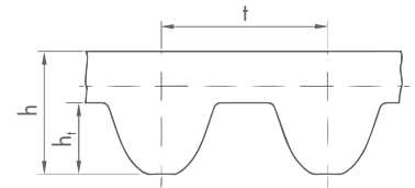
Abbildung 1.3.1: Profil DC
