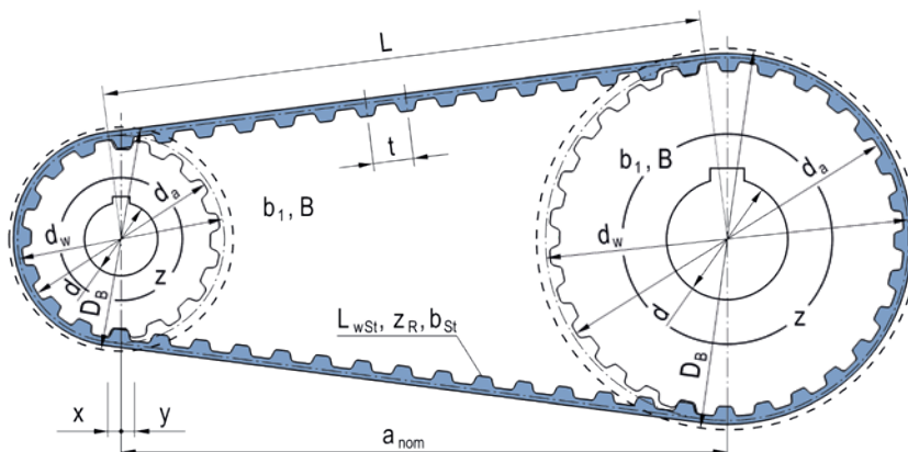
Abbildung 3.1.1: Beispielhafte Getriebegeometrie: Riemen und Scheiben
