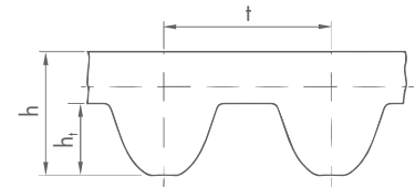
Abbildung 1.3.1: Profil DC
